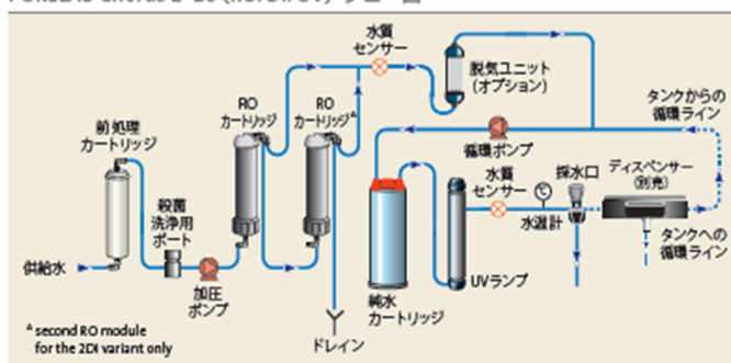
PURELAB Chorus 2+ 20 (RO/DI/UV) フロー図
