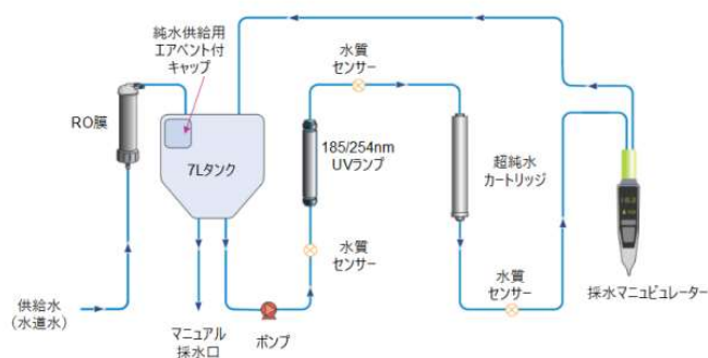
PURELAB flex3 フロー図
